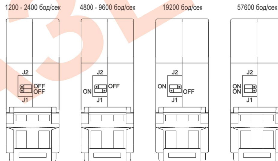
Рис.3 Установка джамперов
