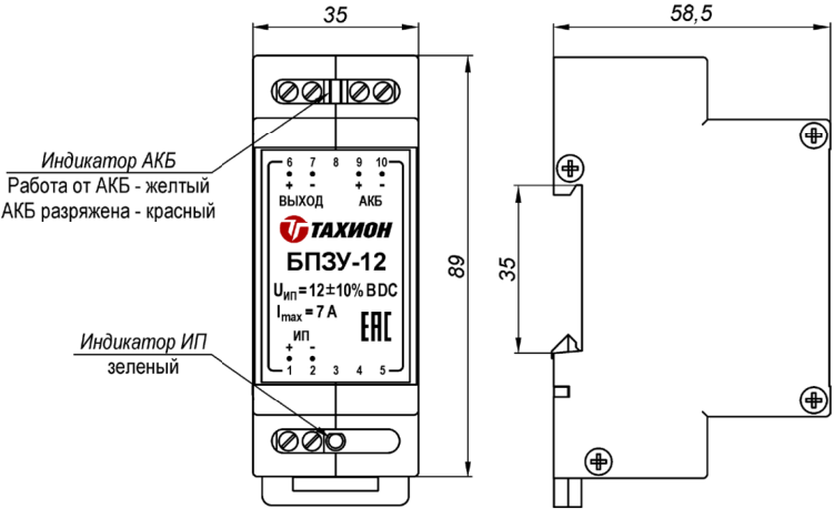
Рис.1 Габаритные размеры
