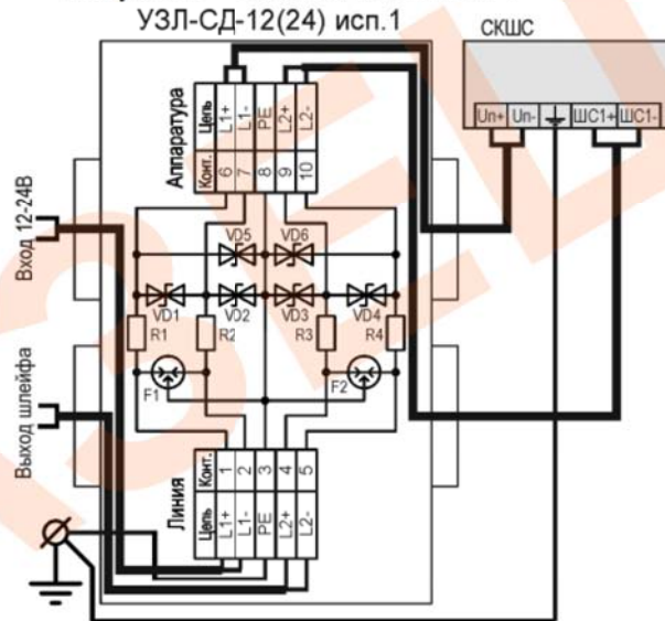
Рисунок 4 – Схема включения 3
