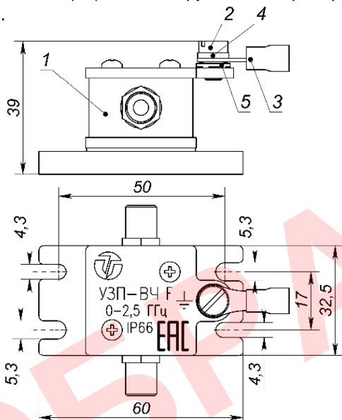
Рисунок 1 – Состав и габаритно-установочные размеры (позиции см. комплект поставки)
