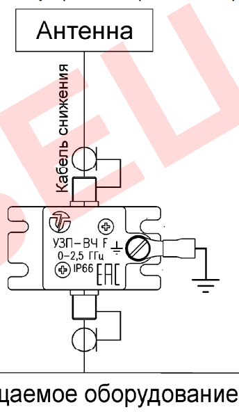
Рисунок 2 – Пример схемы подключения
