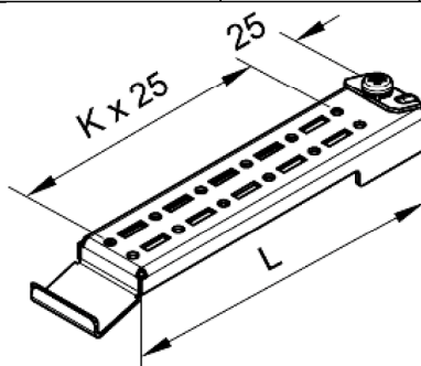
Рисунок 1 – Устройство монтажной шины
