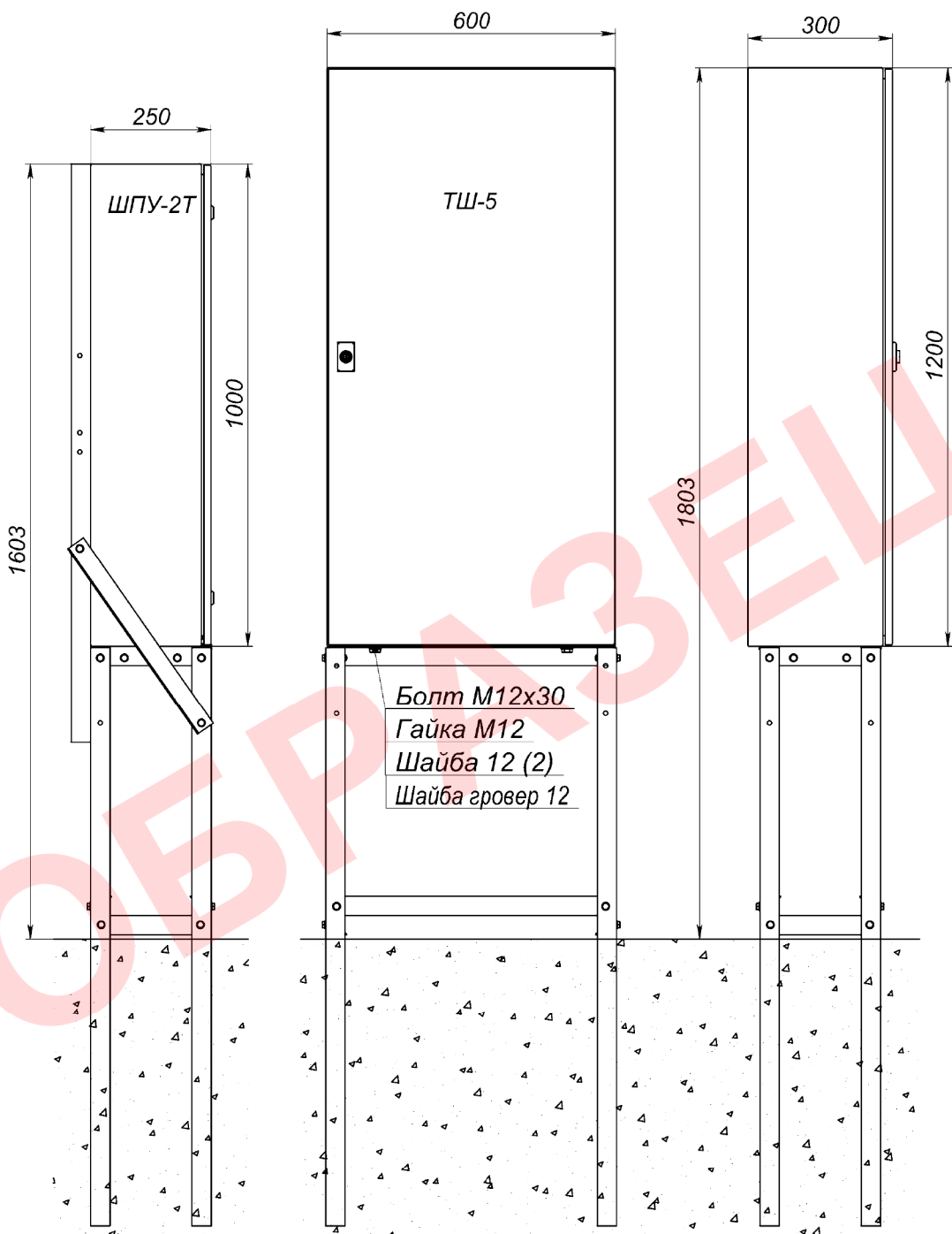
Рисунок 3.2 – Габаритные и установочные размеры основания напольного ОНШ-11.
