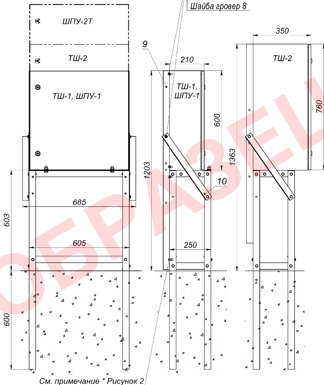
Рисунок 3.1 – Габаритные и установочные размеры основания напольного ОНШ-11.
