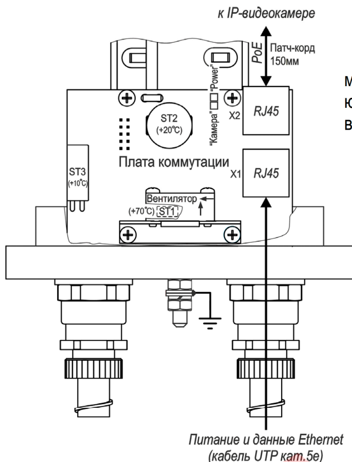
Рисунок 5 – Подключение ТГБ-4Г ТВ Ex IIS-PoE+
