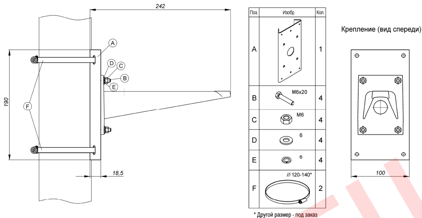
Рисунок 11 – Монтаж кронштейна КС-1 на опору (круглую или квадратную)
