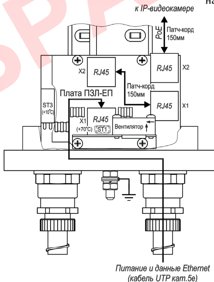
Рисунок 7 – Подключение ТГБ-4Г ТВ Ex IIS-PoE+ с платой ПЗЛ-ЕП
