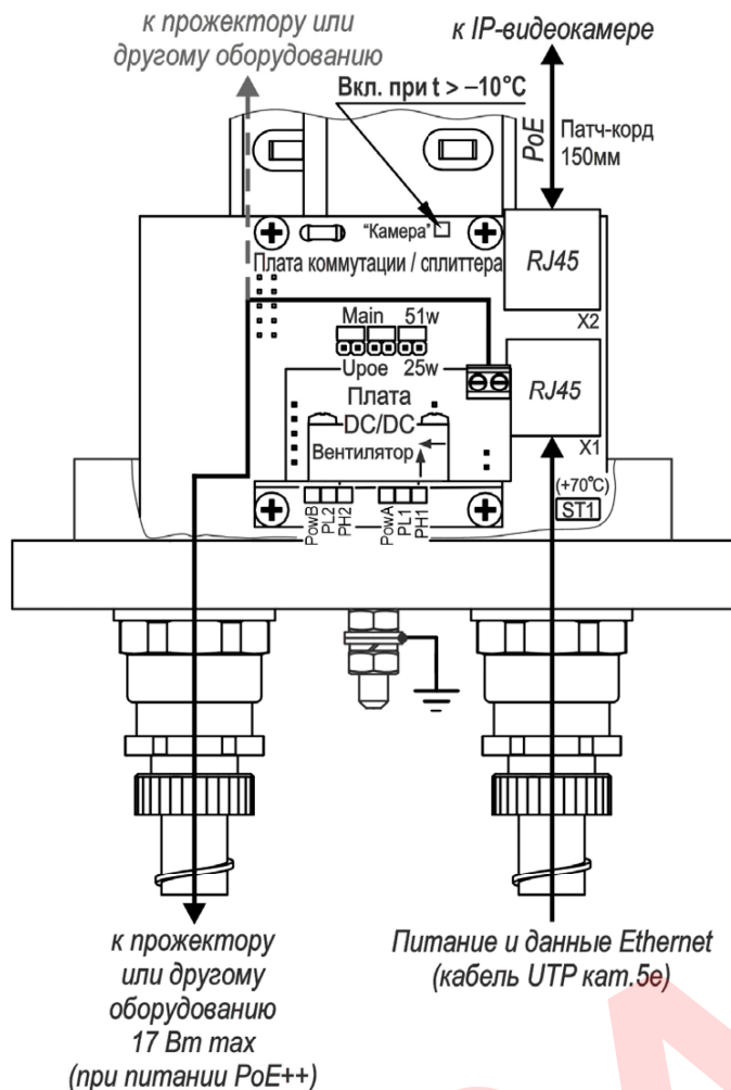
Рисунок 8 – Подключение ТГБ-4Г ТВ Ex IIC-PoE++
