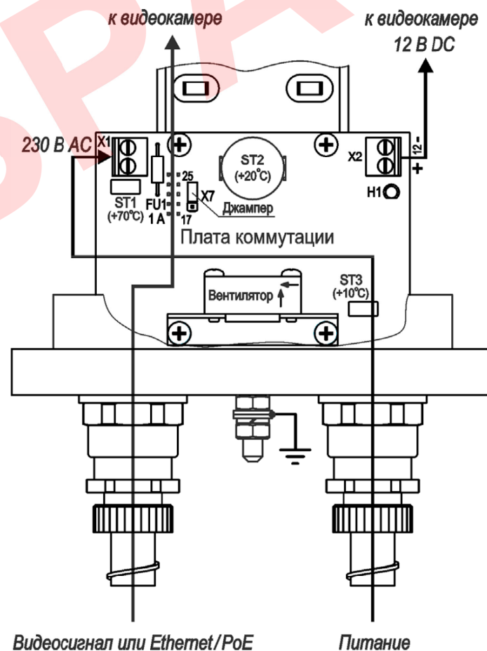
Рисунок 4 – Подключение ТГБ-4Г ТВ Ex IIC-220/12
