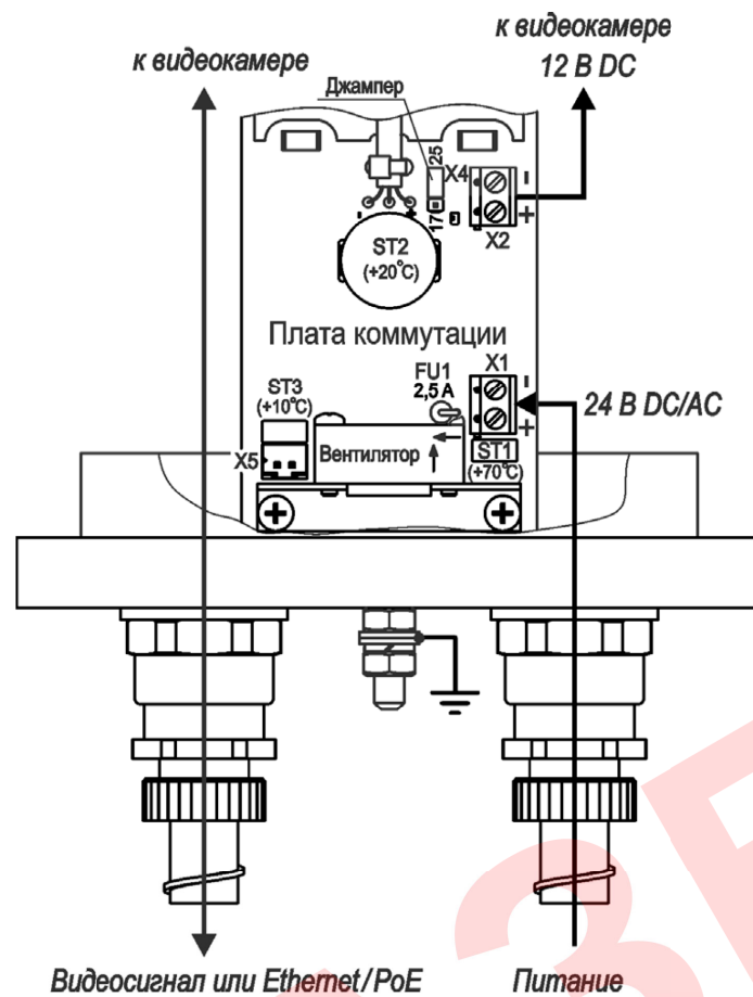
Рисунок 3 – Подключение ТГБ-4Г ТВ Ex IIC-24/12
