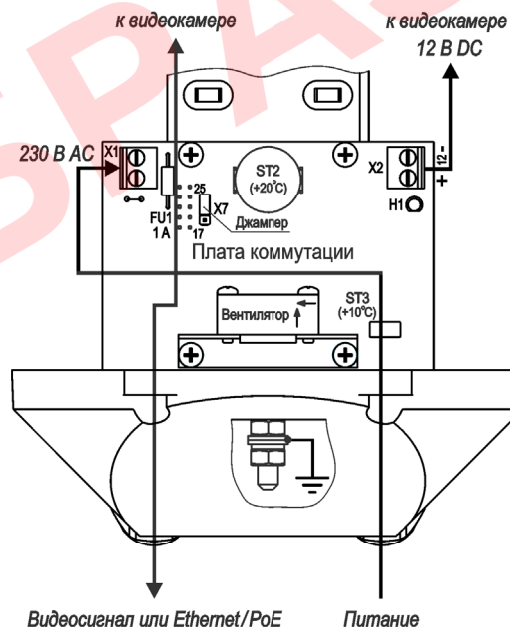
Рисунок 4 – Подключение ТГБ-7 ТВ-220/12
