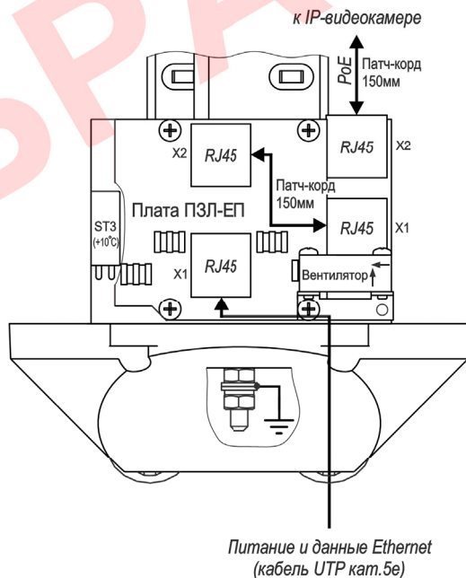
Рисунок 7 – Подключение ТГБ-7 ТВ-PoE+ с платой ПЗЛ-ЕП
