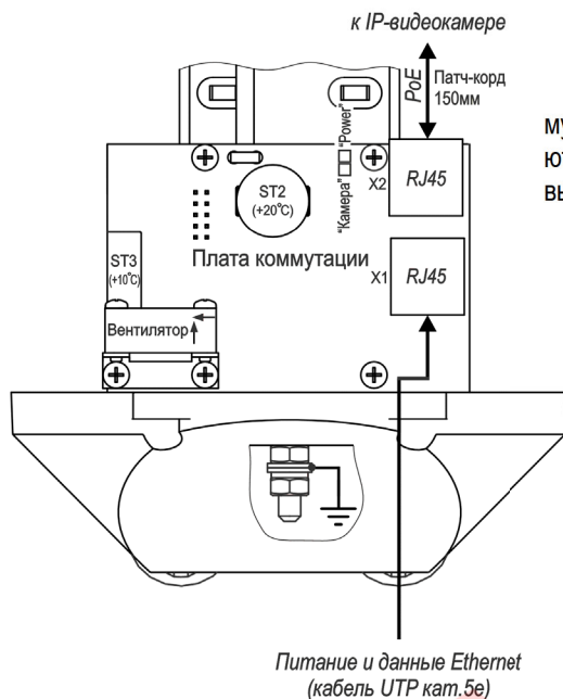
Рисунок 5 – Подключение ТГБ-7 ТВ-PoE+
