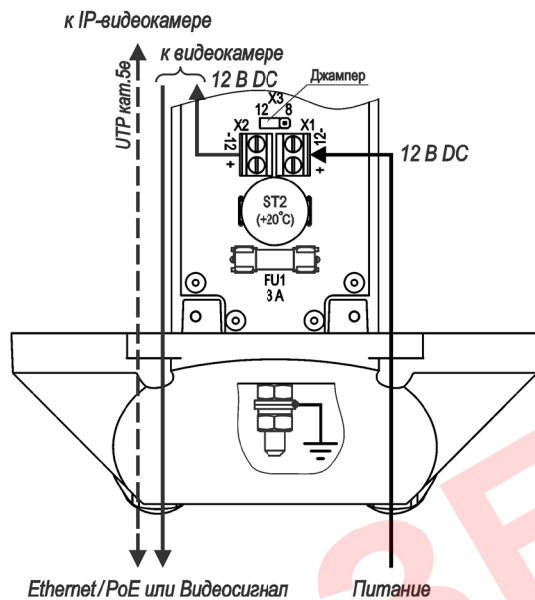
Рисунок 9 – Подключение ТГБ-7 ТВ-12
