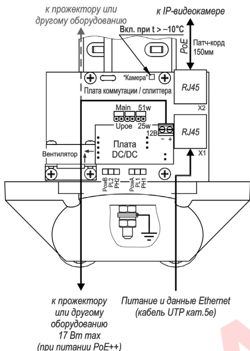
Рисунок 8 – Подключение ТГБ-7 TB-PoE++
