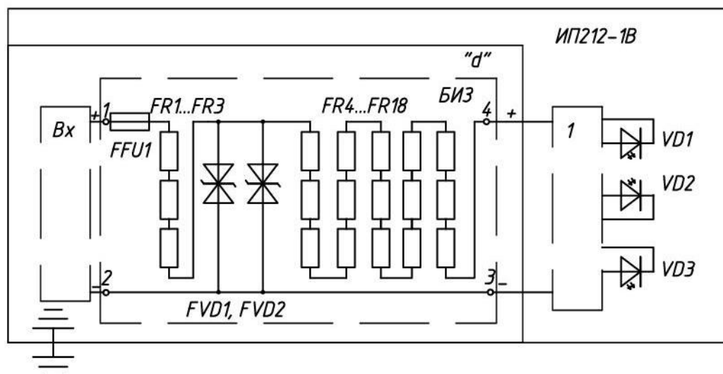
Рисунок Д.1 – Электрическая схема извещателя дымового ИП212-1В
