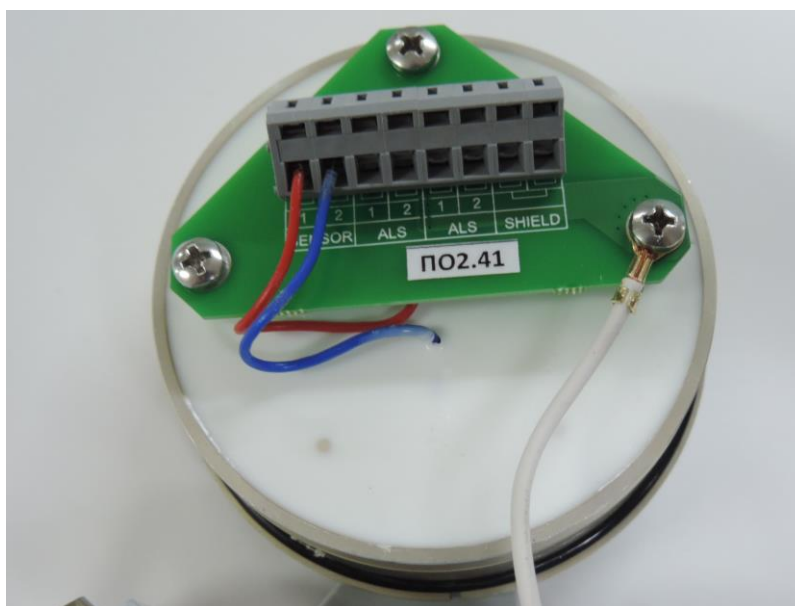
Рисунок А.3 – Вид измерительного блока в сборе сзади. Маркировка версии программного обеспечения на входной плате ИП212-1В-РЗ-А
