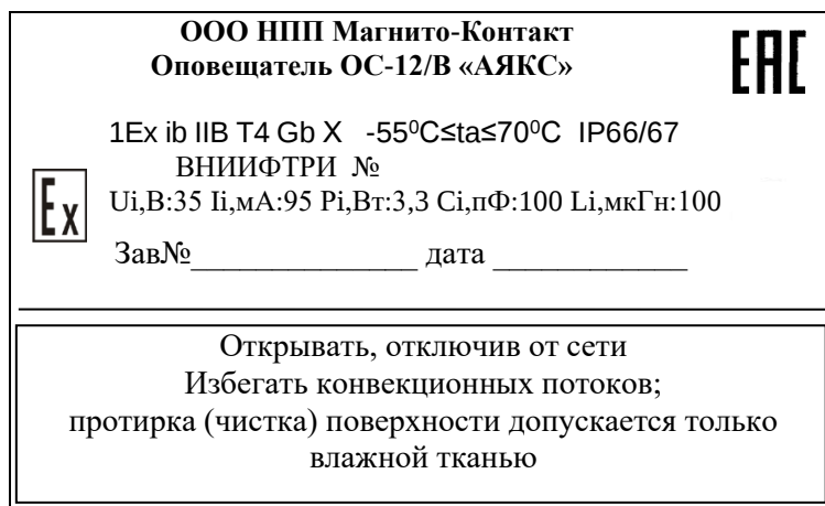
Рис. 1 Маркировка оповещателя ОС-12/В «АЯКС»
