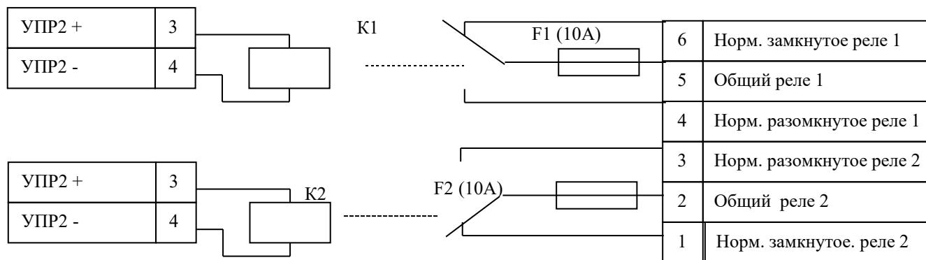
Схема подключения устройства УК-БК-Ех АЯКС
