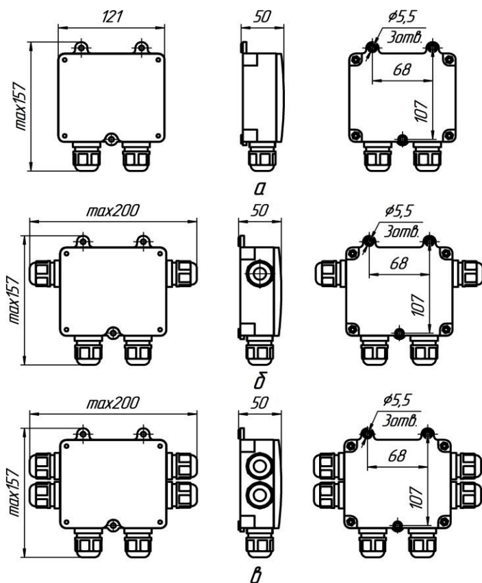
Рис. 1. Установочные и габаритные размеры коробки соединительной.
