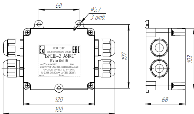
БИСШ-2 АЯКС
