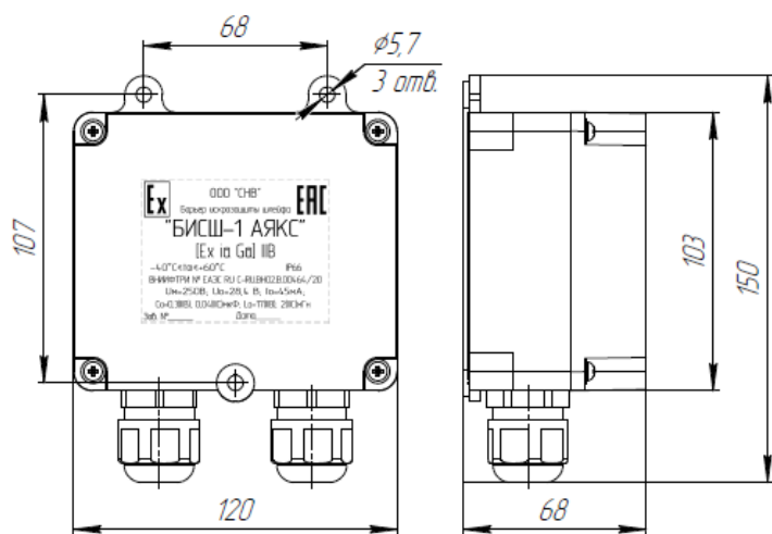
БИСШ-1 АЯКС,
