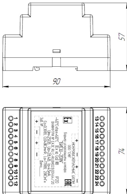
БИСШ-2DIN АЯКС
