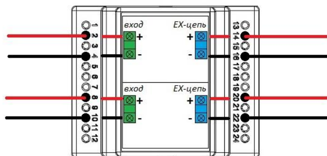
БИСШ-2 АЯКС
