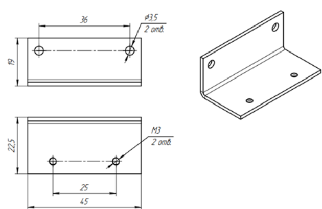
Рис.1. Габаритные и присоединительные размеры КР-29 Эстет Нержавейка
