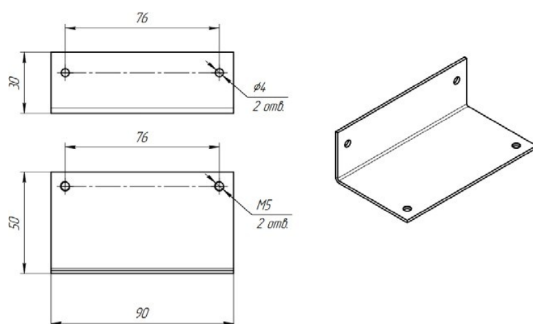
Рис.8 Габаритные и присоединительные размеры кронштейна КР-ДПМ-2 Нержавейка
