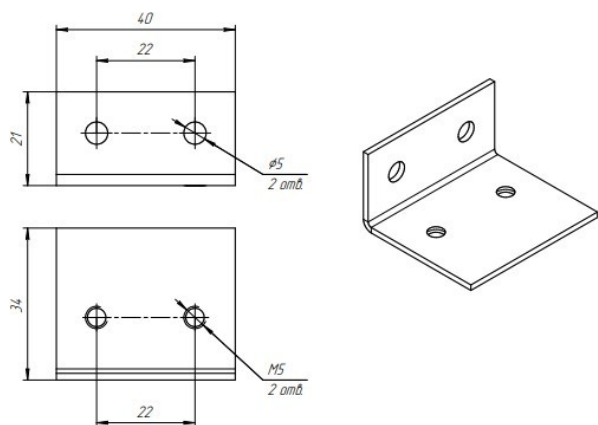
Рис.5 Габаритные и присоединительные размеры кронштейна КР-40 Нержавейка
