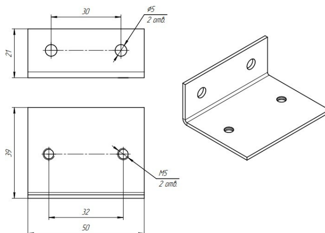
Рис.6 Габаритные и присоединительные размеры кронштейна КР-20/50 Нержавейка
