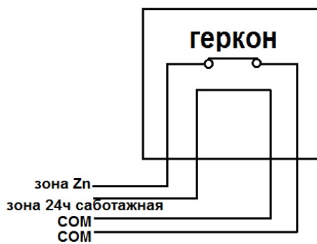
Рис. 3 Примеры подключения датчика положения СК555 к ПКП
