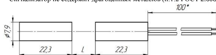
Рис.1 Габаритные размеры.
