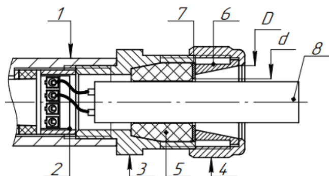
Рис.4.1 открытая прокладка кабеля диам. подключаемого кабеля 6-18мм
