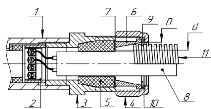
Рис.4.2 установка кабеля в металорукаве диам. подключаемого кабеля 6-18мм
