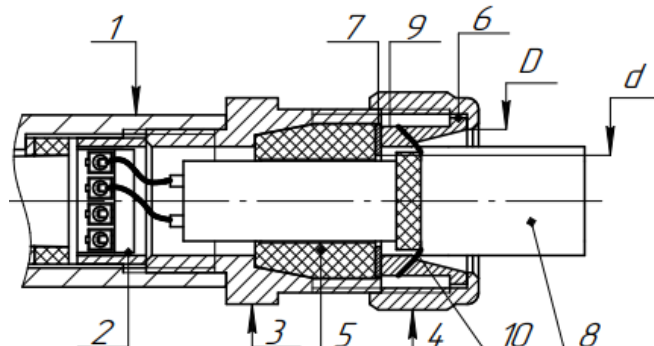
Рис.4.4 установка бронекабеля
