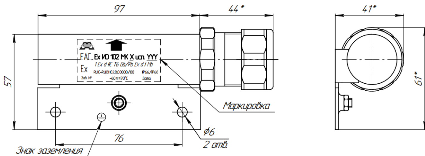
Рис.1 Габаритные и установочные размеры исполнительного блока Ex ИО 102
