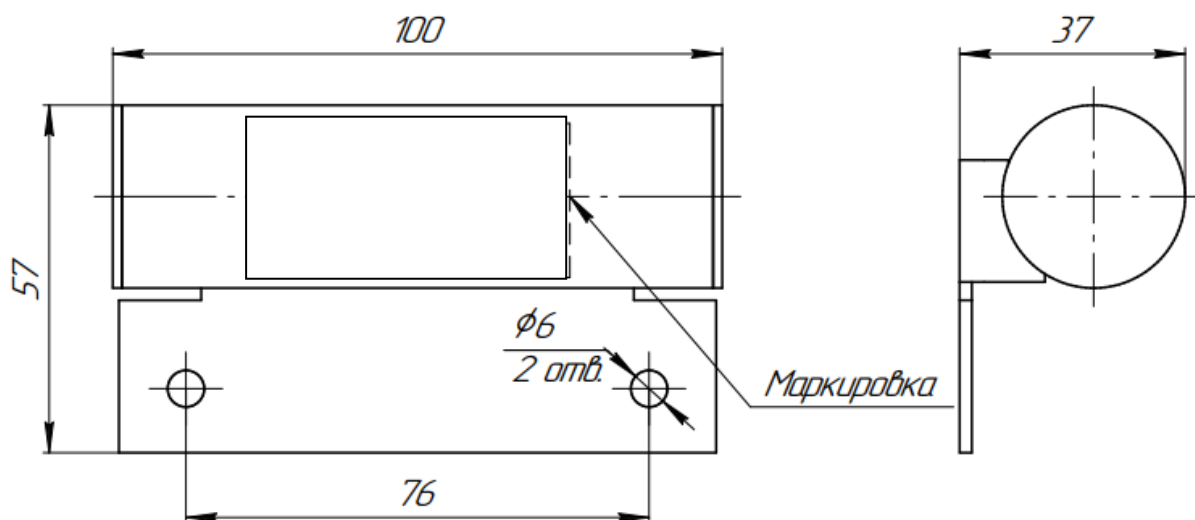
Рис.3 Габаритные и установочные размеры задающего блока Ex ИО 102
