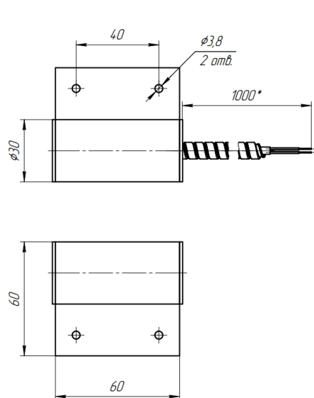
Ри.1. ИО 102-100 с присоединённым кабелем в металлорукаве
