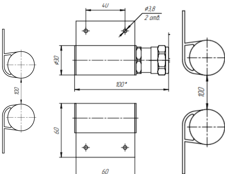
Рис.2 ИО 102-100К с кабельным вводом.
