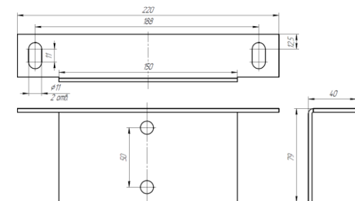
кронштейн К-02
