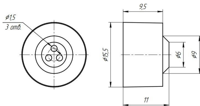
Рис.3 Габаритные размеры уплотнителя типа 3 (под три проводника).
