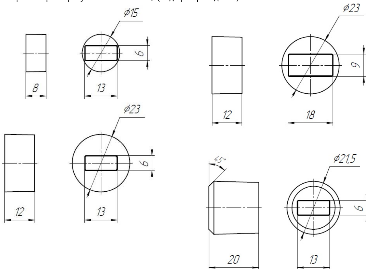
Рис.4. Габаритные размеры уплотнителя типа 4 (под плоский кабель)
