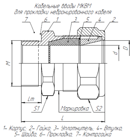
Рис.А1 Кабельные вводы серии Ex МКВМ для открытой прокладки кабеля
