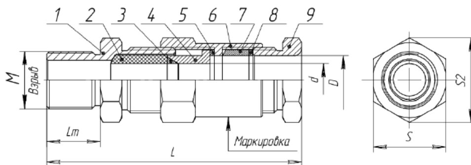
Рис.А4 Кабельные вводы серии Ex MKBM для прокладки кабеля в металлорукаве
