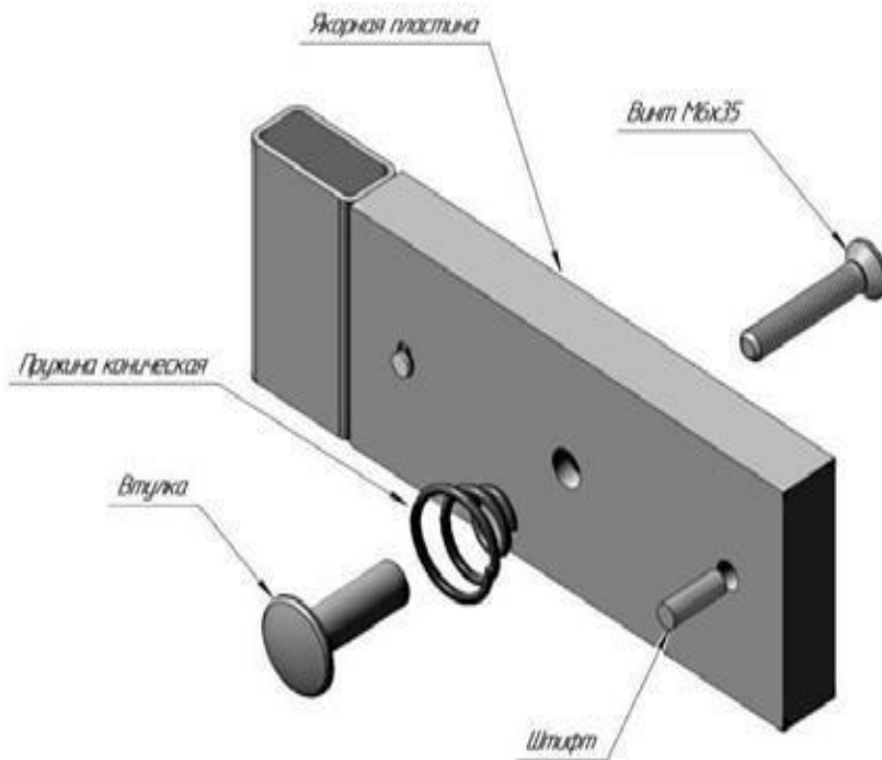
Рис.4 Комплект крепления якоря через сквозное отверстие
