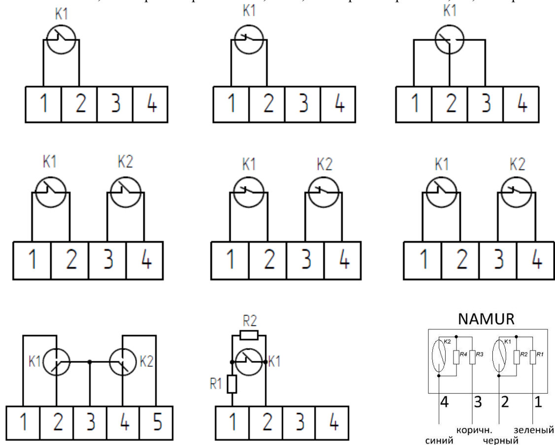
Рис.2 Электрическая схема датчика ДМГ с двумя NO контактами герконов. R1**,R3** - резистор 0.4-2кОм , R2**,R4** - резистор 10кОм, K1, K2 геркон
