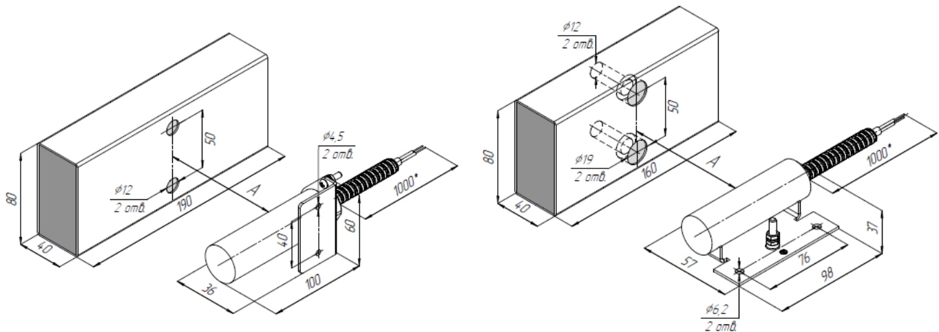
Торцевая крепежная площадка Т (съёмная)
