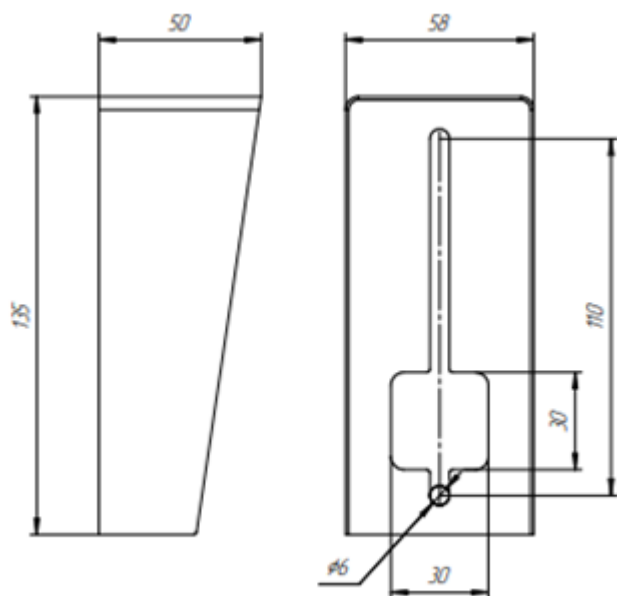
Рис.4 Козырёк защитный 135x58 АЯКС
