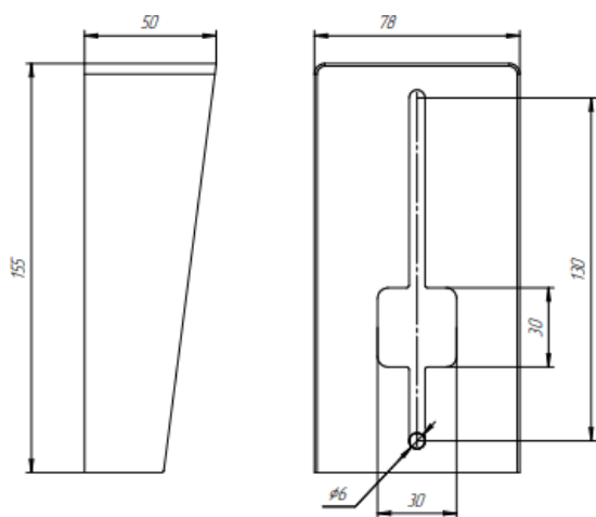
Рис.5. Козырёк защитный 155x78 АЯКС
