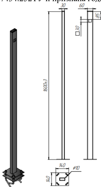
Рис.2 Стойка «Лайт»
