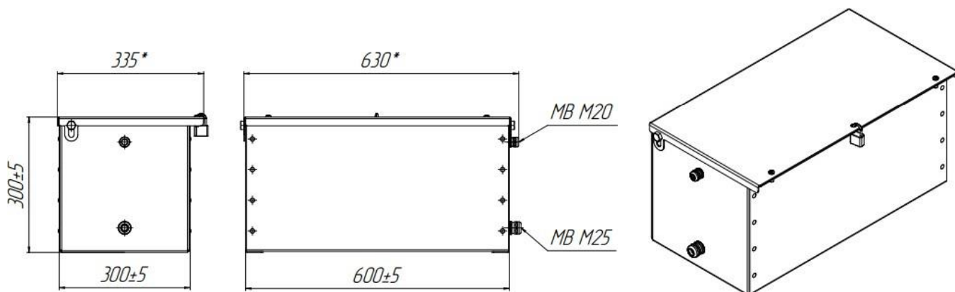
Рис.1 Габаритные размеры Бокса под АКБ.
