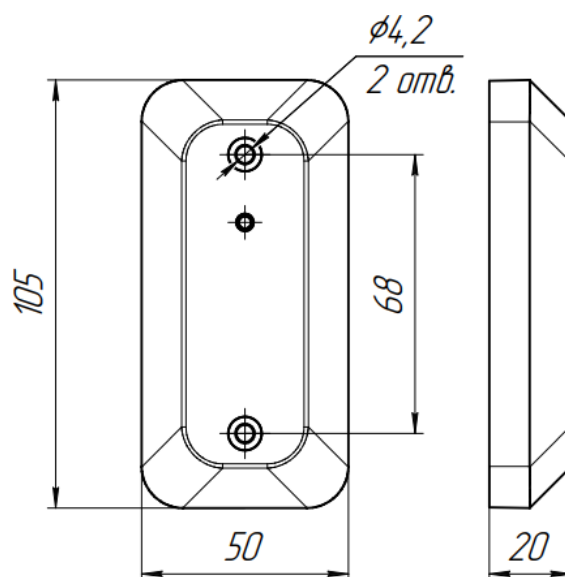
Рис.2 Габаритные размеры Считыватель RD-26 АЯКС без козырька
