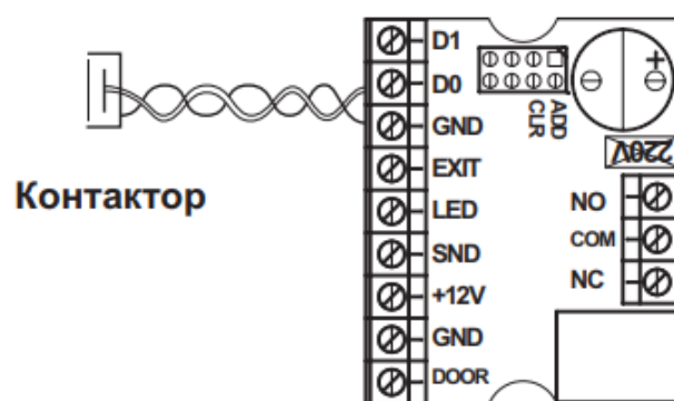
Рис.5 Подключение контактора.
