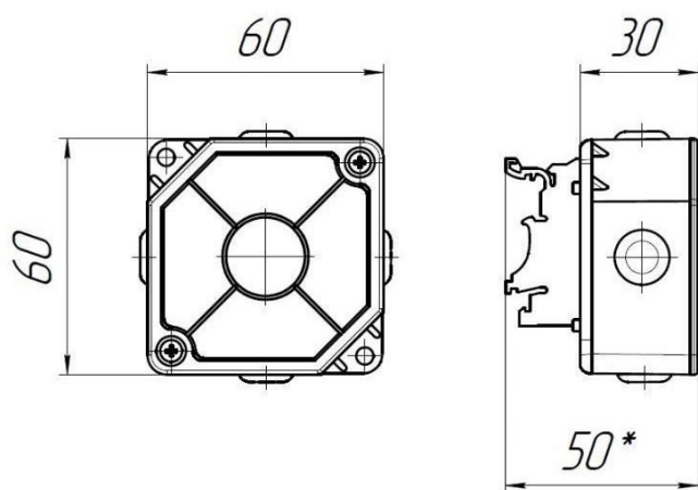
Рис.1 КСП-DIN-5 (60x60x30)
