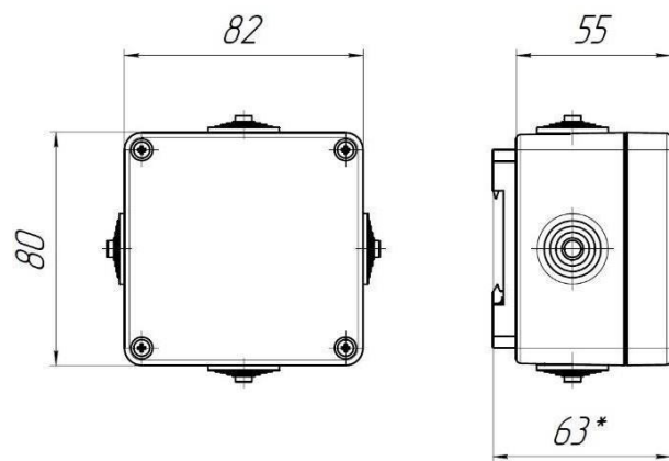
Рис.2 КСП-DIN-7 (82x80x55)
