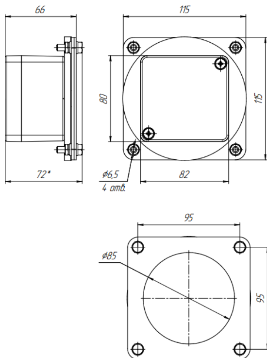
Рис.1 Габаритные и присоединительные размеры. СУМ-1П (пластиковый корпус)
