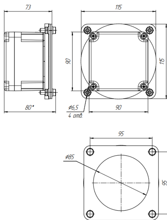
Рис.2 Габаритные и присоединительные размеры СУМ-1М (металлический корпус)
