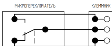
Рис. 3 Схема электрического соединения
