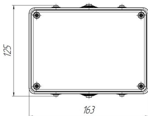
Рис.3 КСП с DIN-рейкой (163x125x86)
