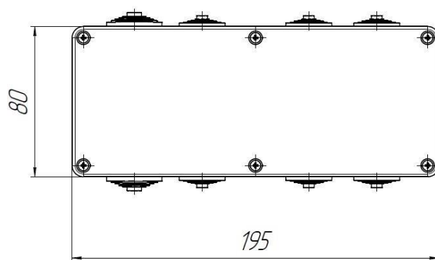
Рис.4 КСП с DIN-рейкой (195x80x75)
