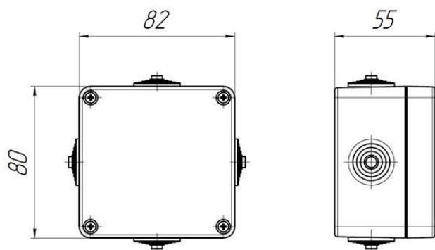
Рис.1 КСП с DIN-рейкой (82x80x55)
