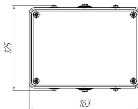
Рис.2 КСП с DIN-рейкой (163x125x66)
