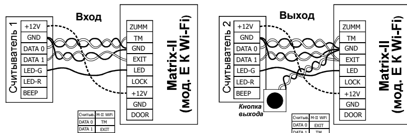
Рис.5 Подключение внешних считывателей по протоколу Wiegand
