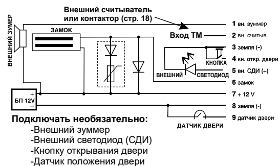
Рис. 3 Подключение внешних устройств
