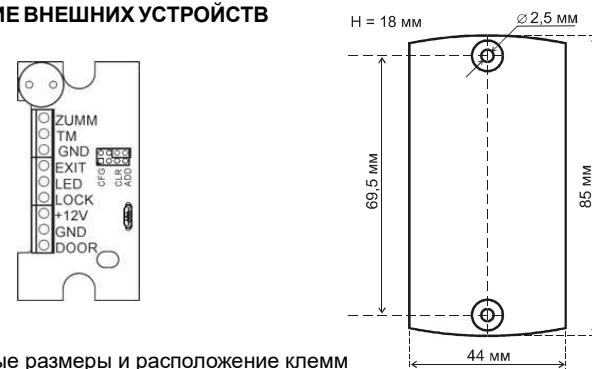
Рис.1 Габаритные размеры и расположение клемм
