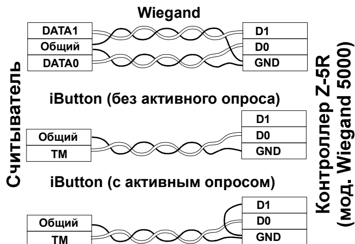
Рис.3 Варианты подключения внешних считывателей
