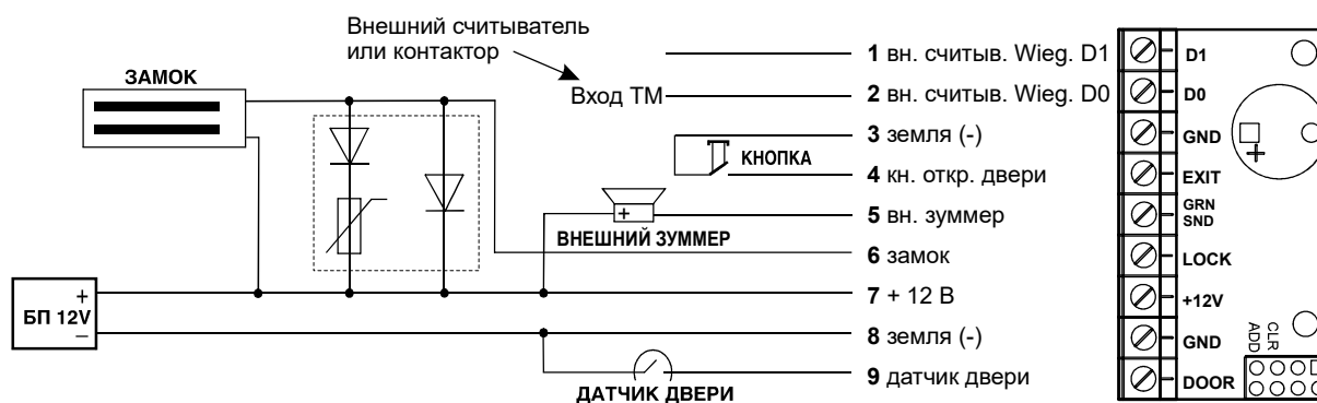
Рис.5 Схема подключения внешних устройств
