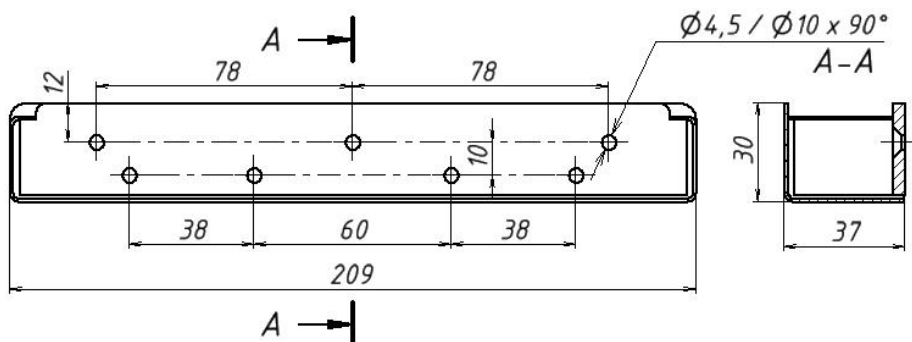
Рисунок 2 – Габаритно-установочные размеры комплекта МК 700S
