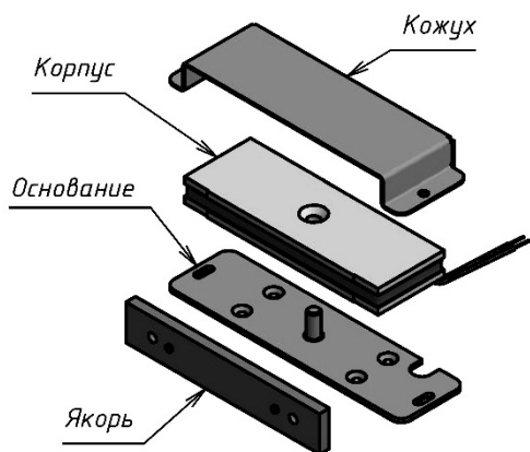
Рисунок 1 – Комплект поставки
