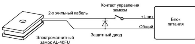
Рисунок 5 – Схема подключения замка
