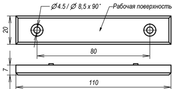
Рисунок 3 – Якорь
