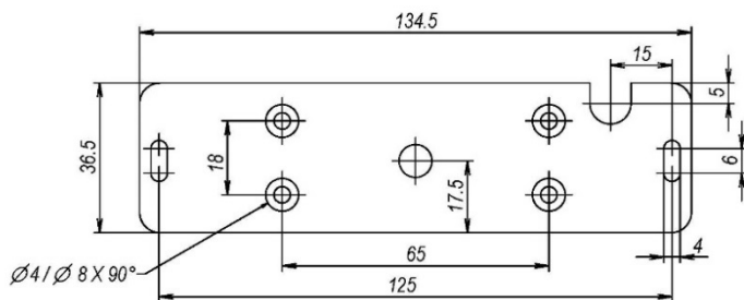
Рисунок 4 – Основание
