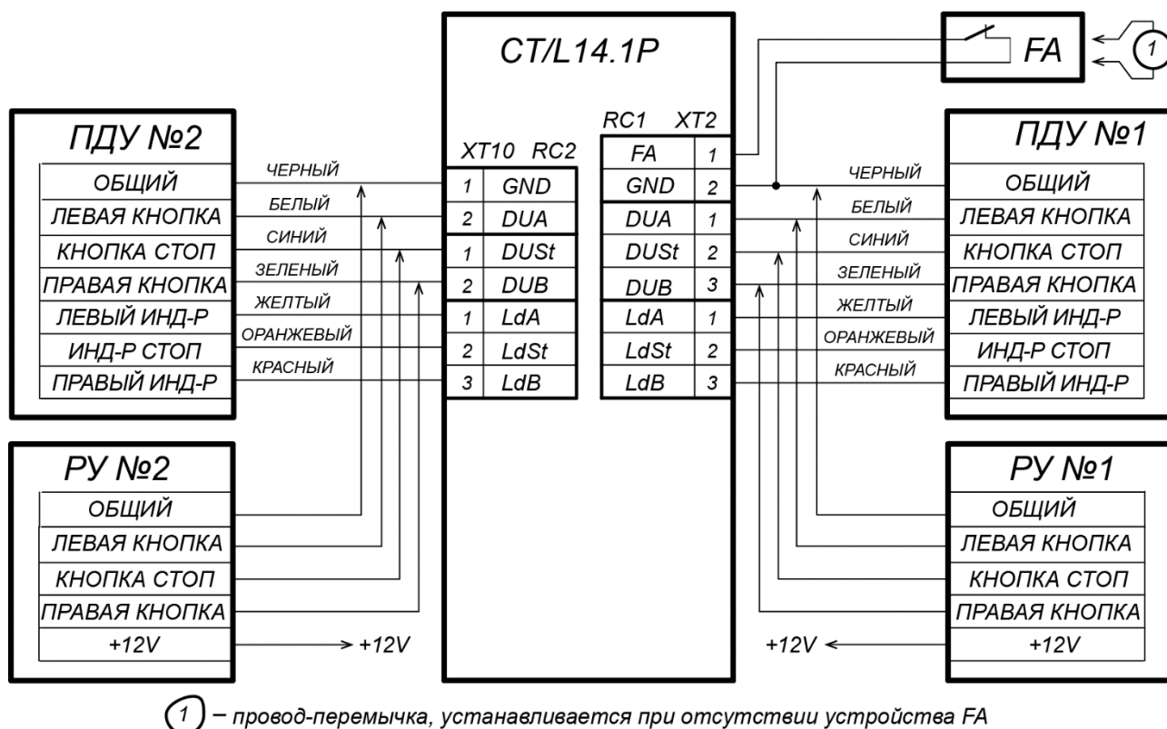
Рисунок 12. Схема подключения ПДУ или устройства РУ для вариантов конфигурации «Контроллер для управления турникетом» и «Контроллер АТП»
