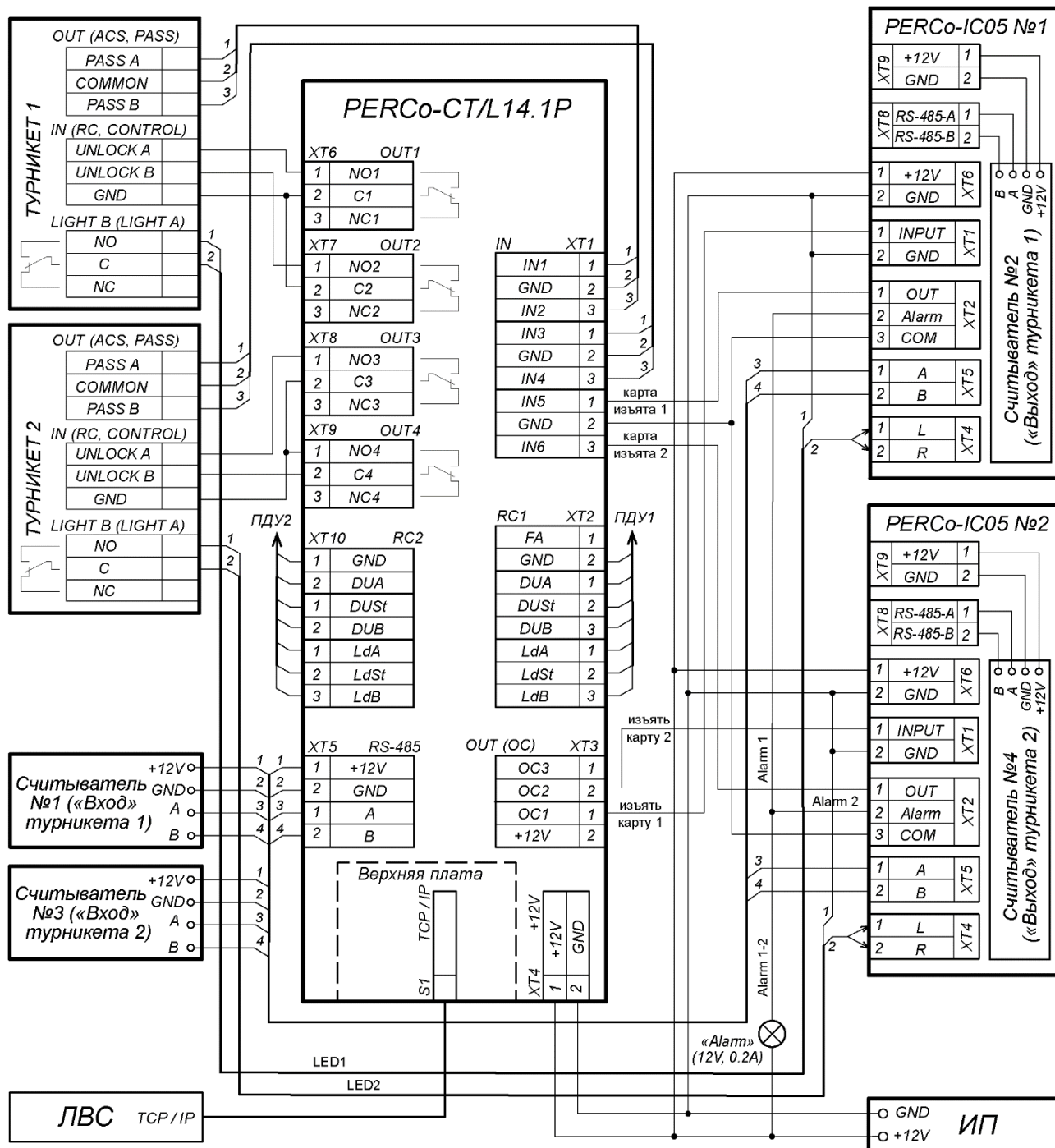
Рисунок 17. Схема подключения двух турникетов с картоприемниками PERCo-IC05
