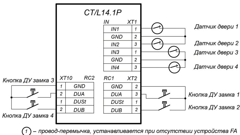
Рисунок 6. Схема подключений кнопок ДУ и датчиков двери
