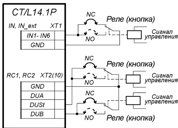
Управление от реле или кнопки
