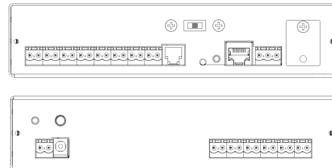
Рис. 2. Вид передней и задней панелей УМА-5И(С), общий.
