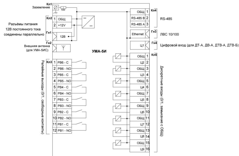
Рис. 1. Графическое отображение УМА-5И на электрической схеме.
