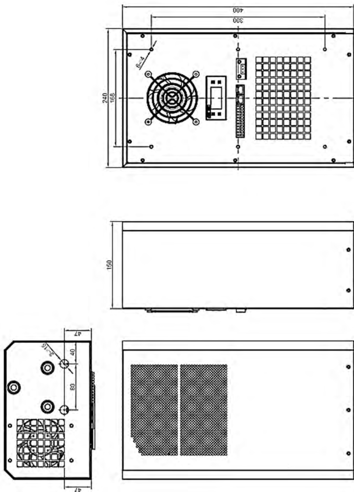
Рисунок 2. Габариты НКА-300-48.
