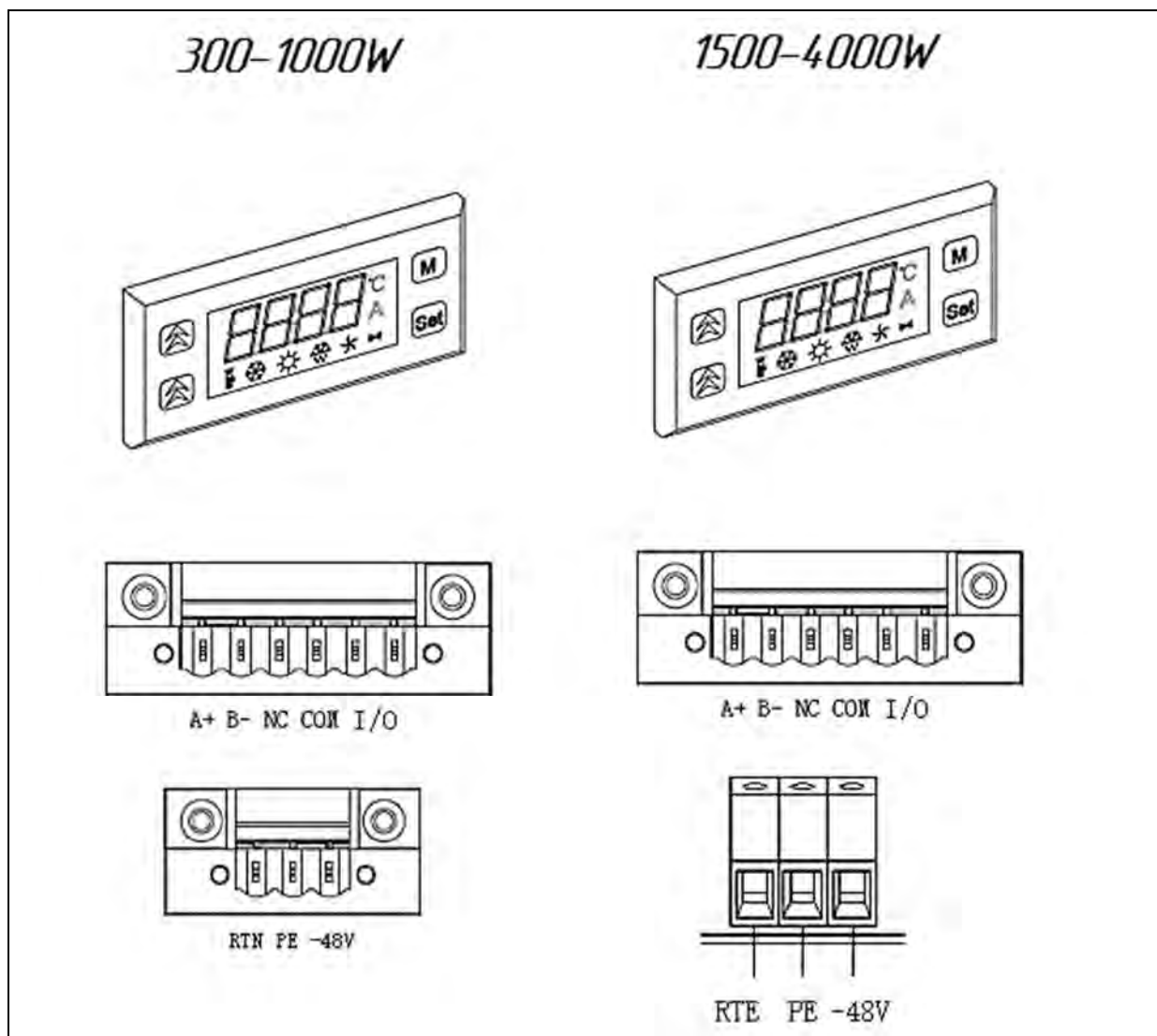
Рисунок 10. Схема подключения.
