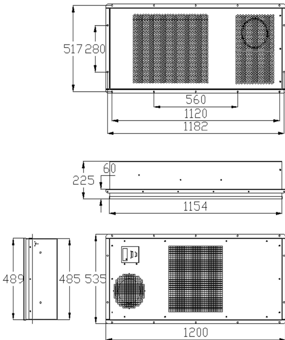
Рисунок 6. Габариты НКА-2500-48 и НКА-3000-48.
