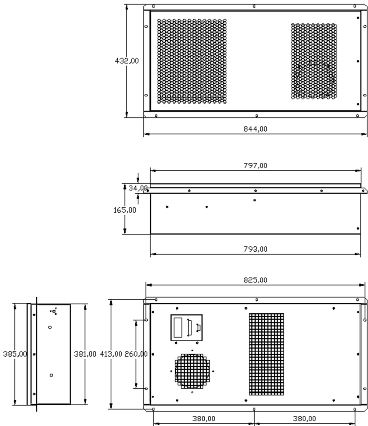
Рисунок 4. Габариты НКА-1000-48.
