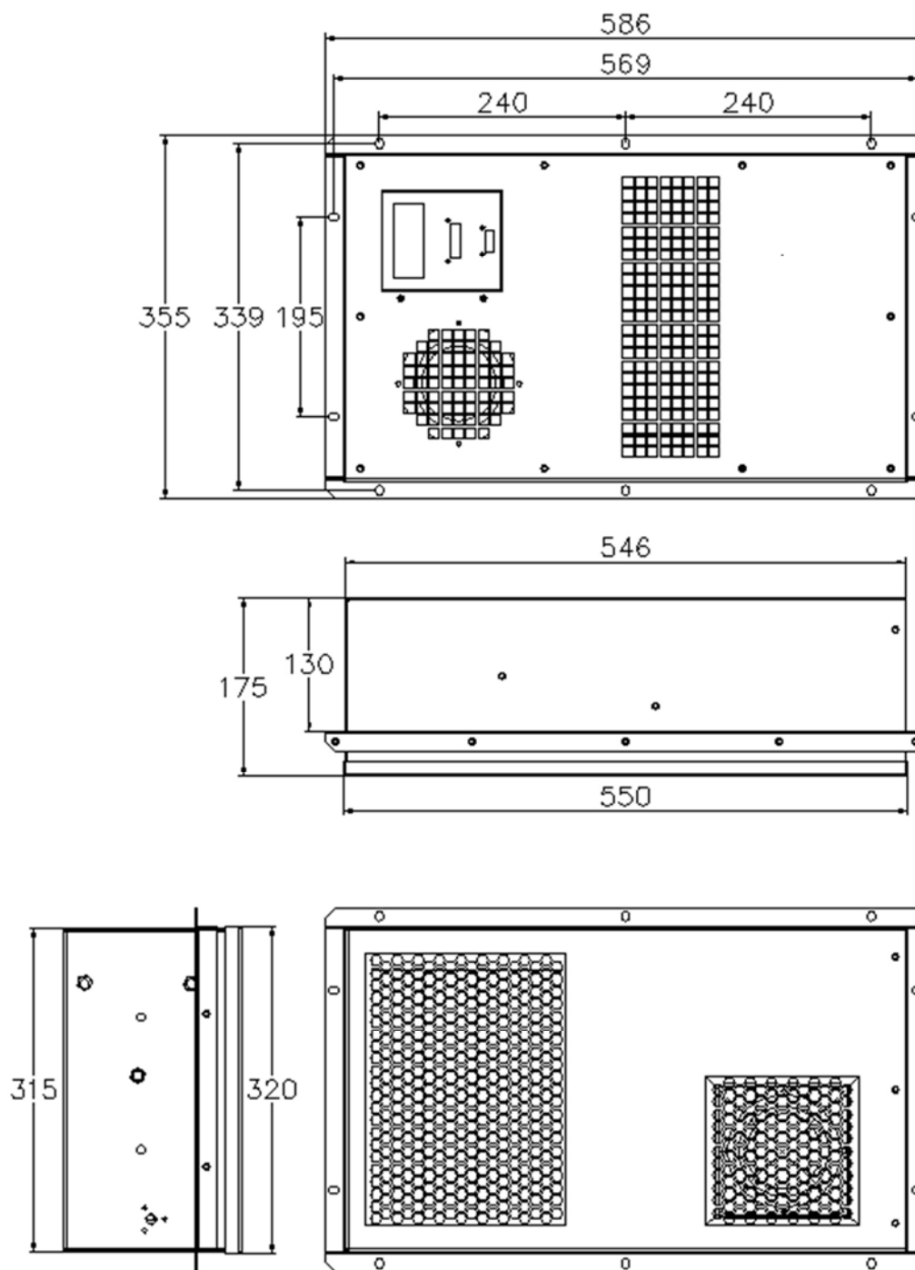
Рисунок 3. Габариты НКА-500-48.
