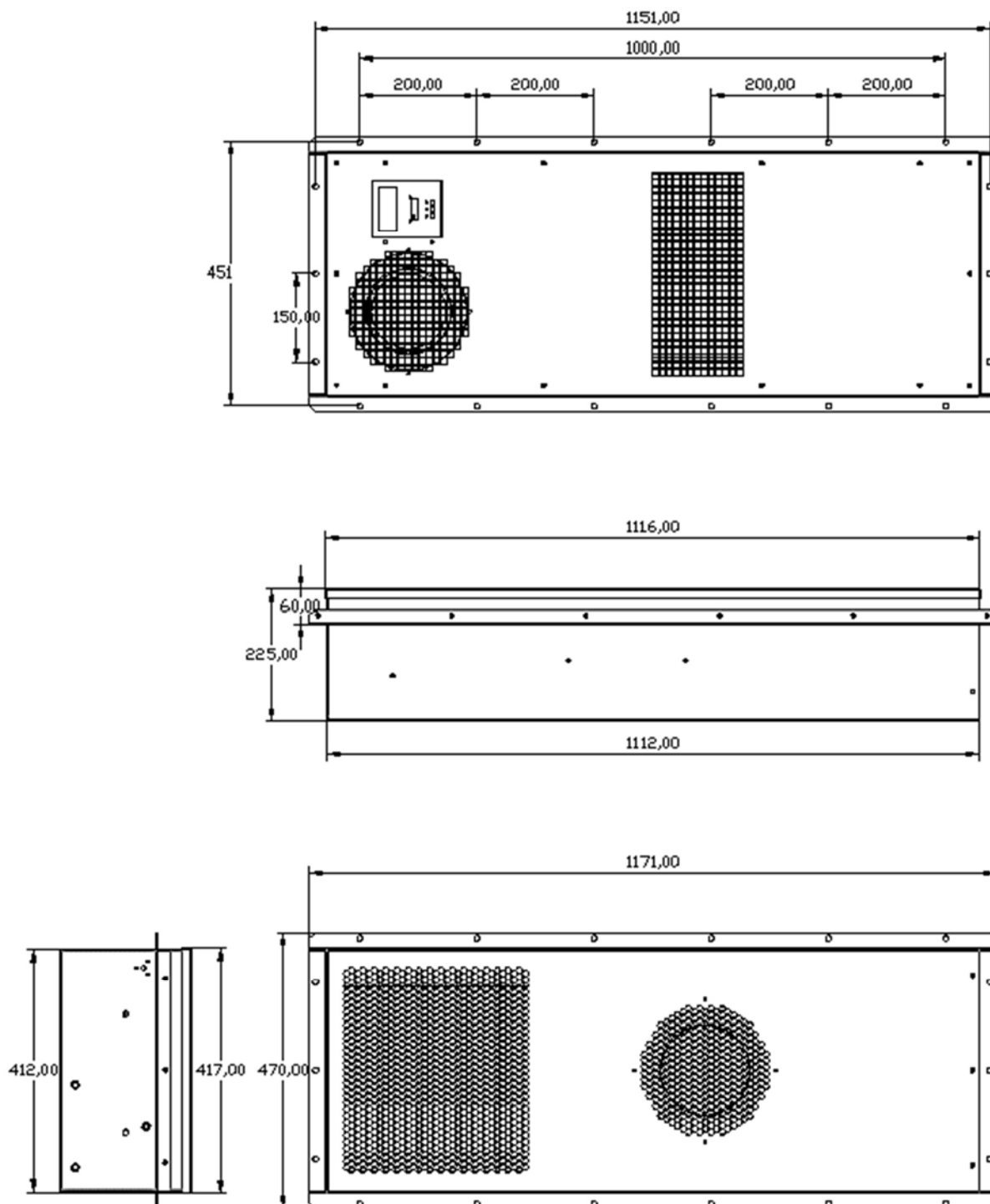
Рисунок 5. Габариты НКА-1500-48 и НКА-2000-48.
