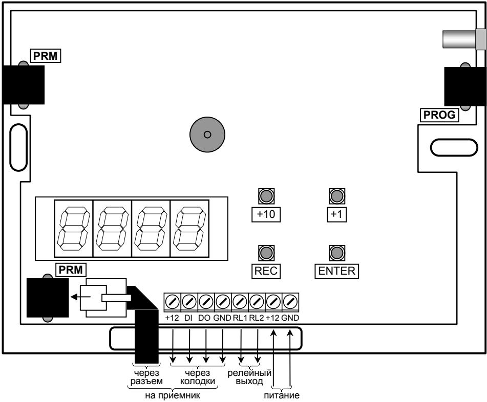
Рис. 4. Монтажная схема пульта при внутреннем подключении
