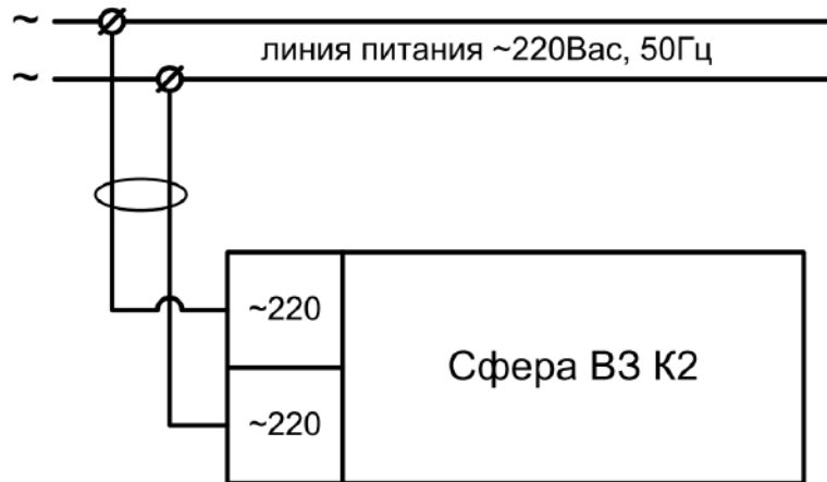
Рис. 2 Схема подключения
